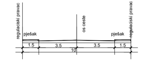
KARAKTERISTIČNI POPREČNI PRESJEK A-A M 1:200
