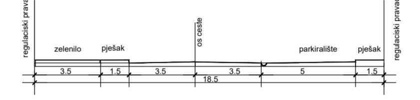
KARAKTERISTIČNI POPREČNI PRESJEK B-B
